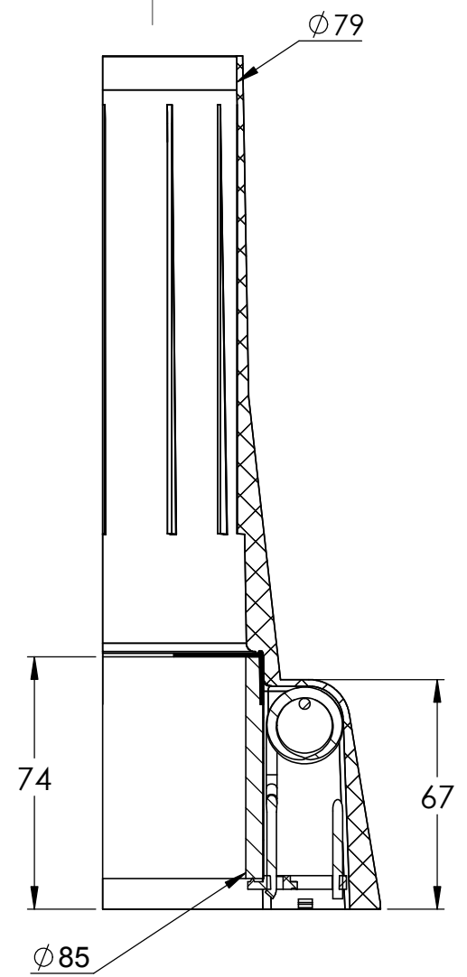
SECTION G-G SCALE 1 : 2
