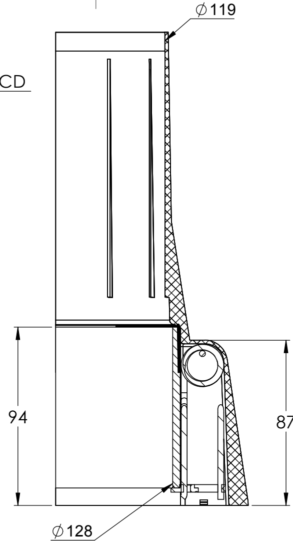
SECTION G-G SCALE 1 : 2
